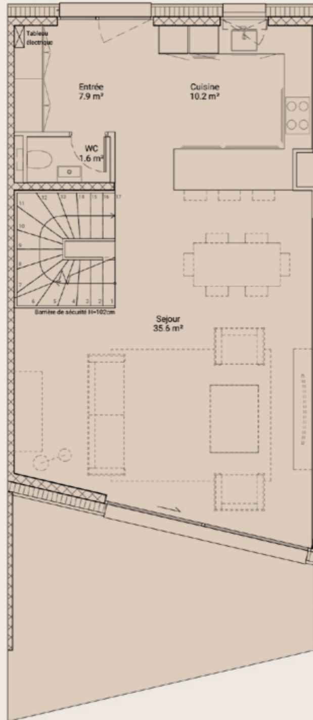
REZ-DE-CHAUSSÉE (70.5 M 2 )
