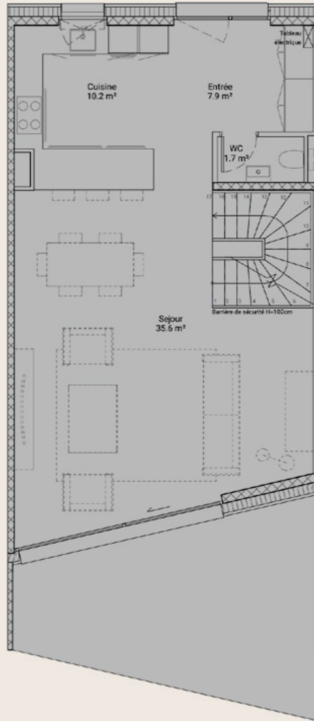
REZ-DE-CHAUSSÉE (70.5 M 2 )
