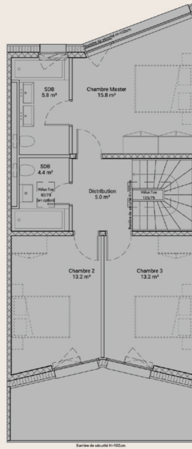
ÉTAGE (75.9 M 2 )
